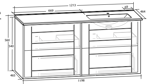
MÖBELPAKET 120, MED 4 LÅDOR OCH ENKEL HO TILL HÖGER
