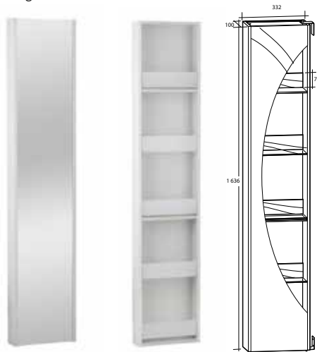
ARIELLA SPEGELHÖGSKÅP 1 spegel, 5 fack
